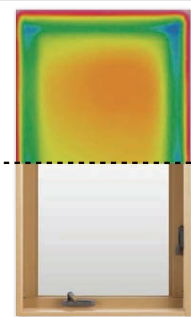
【一般複層ガラス】
